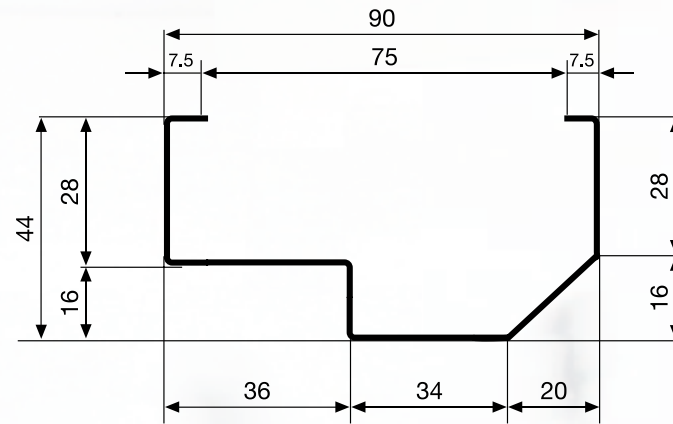
MARCO DE 70 MM PERFIL MARCO - DIMENSIONES FRAME DOOR PROFILE PROFIL CADRE PORTE
